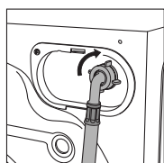
Vízbevezető nyílás a jobb felső oldalon.
