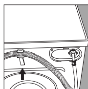
Kampó, ha az elvezető cső 60 cm alatti magasságban végződik.
