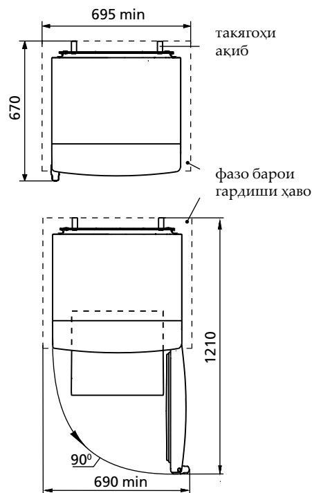
Расми 2 – Яхдон (намуди болої)
