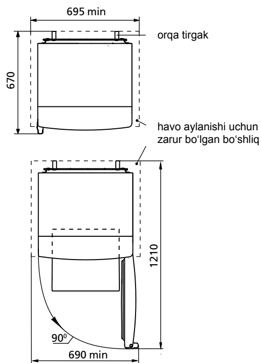
2 rasm – Sovutgich (tepadan ko'rinish)
