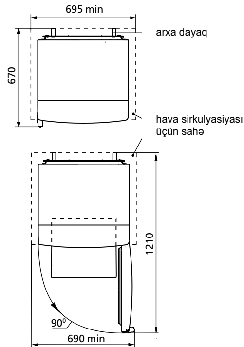
Şəkil 2 – Soyuducu (yuxarıdan görünüş)
