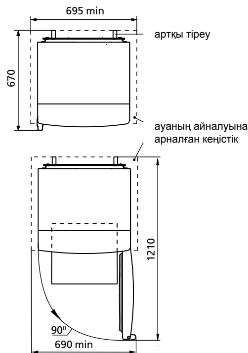
2 сурет – Тоңазытқыш (үстінен қарағанда)
