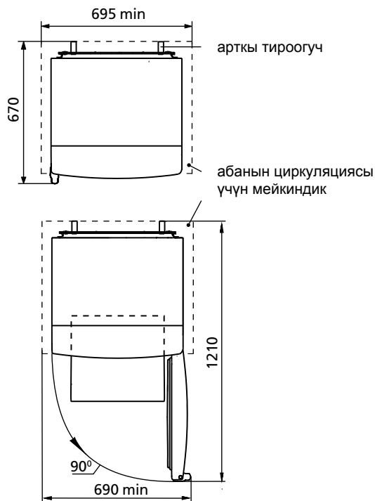
Сурот 2 – Муздаткыч (устунон корунушу)
