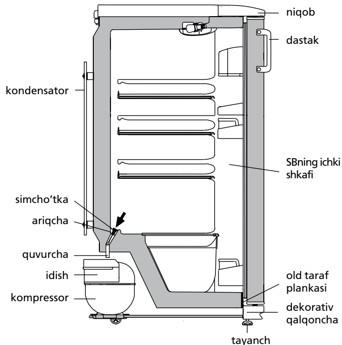
4 rasmi – SBdan erigan suvni oziqlash sxemasi
