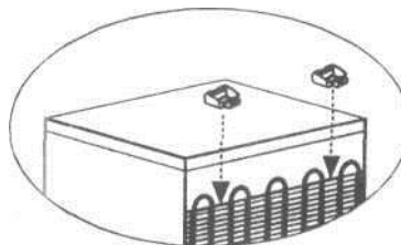
Рис.6 Схема установки задних упоров
