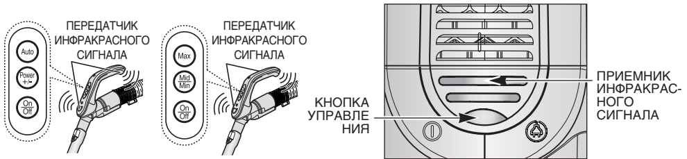
РУЧКА УПРАВЛЕНИЯ
